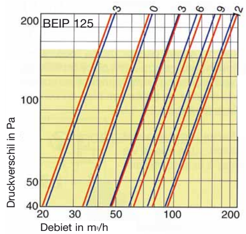
Nevenstaande grafieken geven de druk-debiet curven weer voor de roosters BEIP De cijfers boven de grafiek, geven de regeling weer R in mm.
